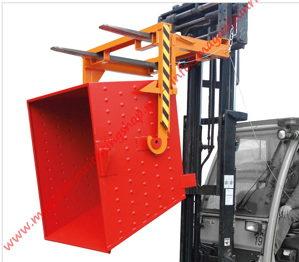
Type BSK-N in kiepstand
