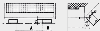
Aanslagpunten voor PSA (persoonlijke beschermuitrusting)
