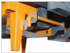
Afglijdbeveiliging middels boutvergrendeling voor de heftruck
