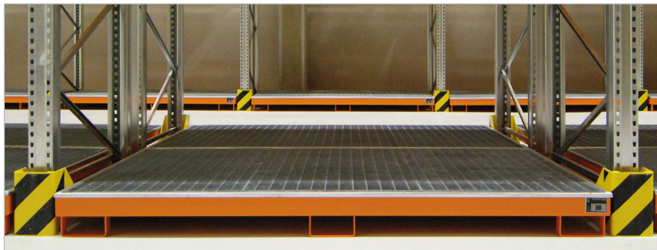
Stelling opvanbak type RW-GR 2700-1 PE
