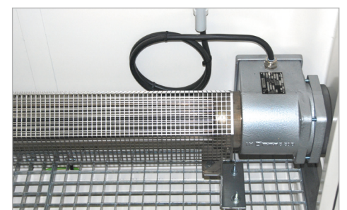
Ex-verwarming, elektrisch
