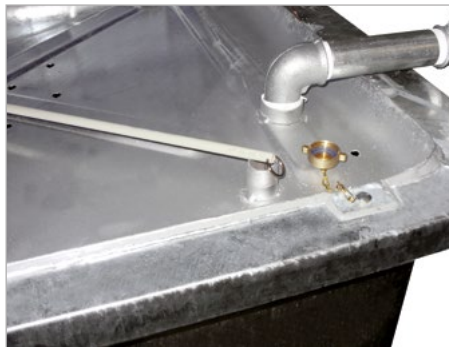
Peilstok voor vulstandcontrole
