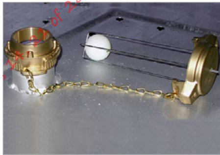
Vulstandmeter / overloopbeveiliging
