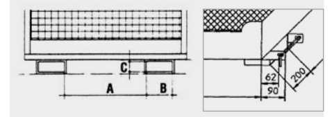
Inrijdkoker-binnenmaten (mm)
