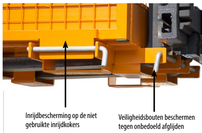
Beveiligingen van de neerklapbare beschermroosters
